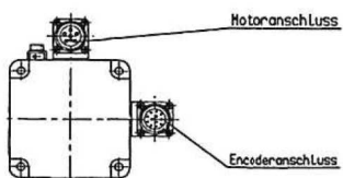
Ansicht A (nur Schrittmotor)
